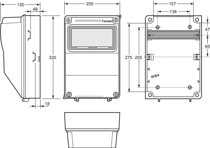
Caja ciega / Blind box - Ref. Item 3958
