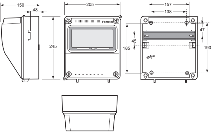
Caja ciega / Blind box - Ref. Item 3958
