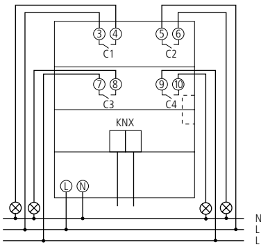
RMG 4 I KNX
