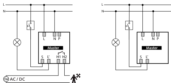
theRonda P360-101 M UP
