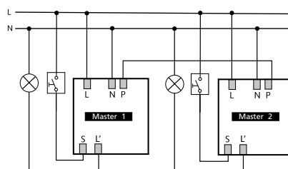
theRonda P360-100 M UP, theRonda P360 Slave UP
