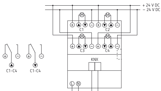
JMG 4 T 24V KNX, JM 4 T 24V KNX
