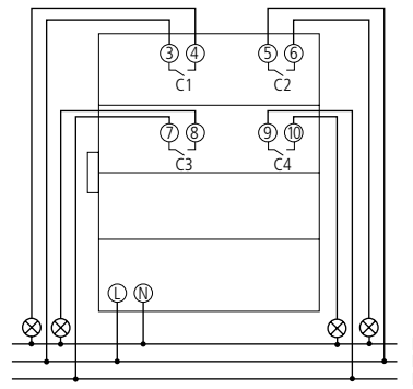
RME 4 I KNX
