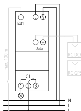
TR 611 top3 RC
