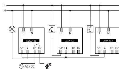
LUXA 103 S360-101, en conexión en paralelo con pulsadores
