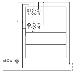
DME 2 T KNX
