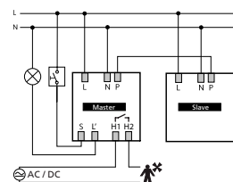
thePrema P360-101 E, thePrema P360 Slave E
