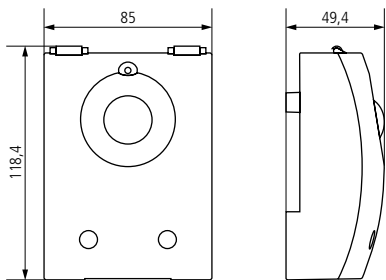
Placa adaptadora LUNA star ↳ N.º art.: 9070486 Detalles en la página 309
