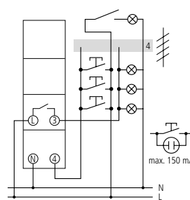
ELPA 6 plus, ELPA 7
